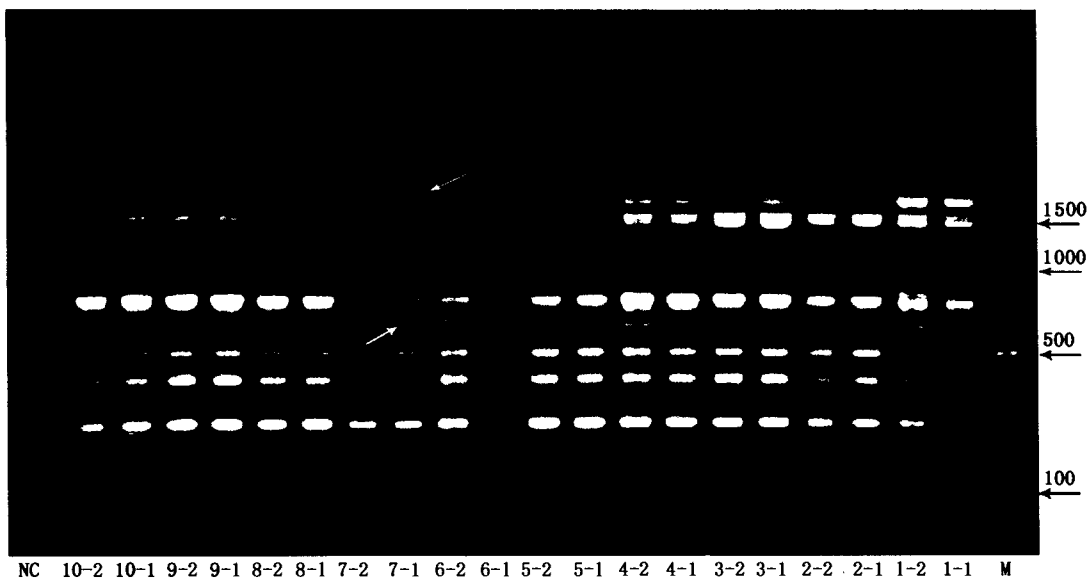
图 1 引物 BA0055 对全部样品的 RAPD 扩增
