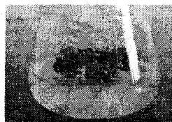
图 2 在 10 号培养基上分化的丛生芽
