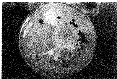
图2 试管苗生根
