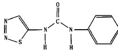
图 1 TDZ 分子结构式
